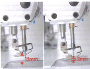
Acionamento do calcador por motor de passo.
