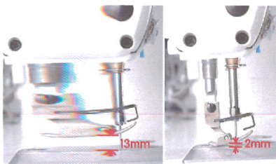
Acionamento do calçador digital (sem solenoide)
