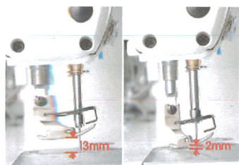
Acionamento do calcador por motor de passo.
