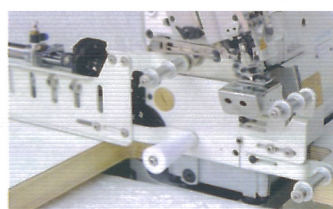
Opcional: rolete (fixo ou móvel) para aplicação de elástico
