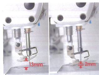
Acionamento do calcador digital (sem solenoide)
